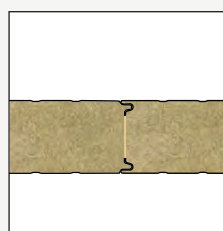
Particolare giunzione
