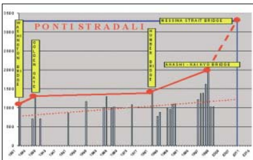
Fig. 2 - Evoluzione dei ponti stradali
